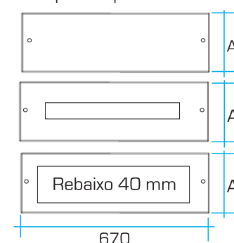
Espelhos aparafusados
